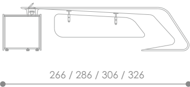
СТОЛ ПИСЬМЕННЫЙ С БОКОВОЙ ТУМБОЙ [BJD-2622W-R/L] Ш: 266 / Г: 220 / В: 76 [BJD-2822W-R/L] Ш: 286 / Г: 220 / В: 76
